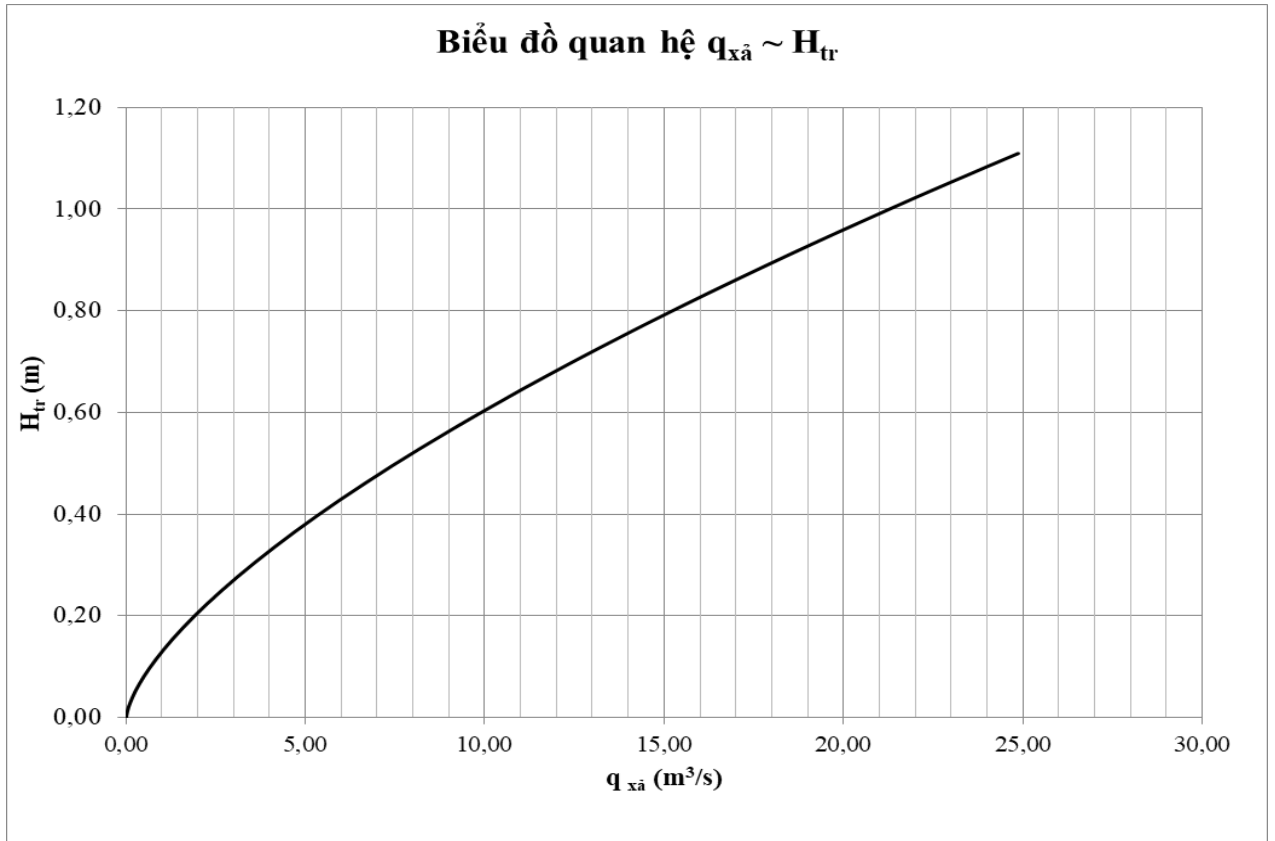
Hình 1: Biểu đồ quan hệ ( Q_{\text{xã}} \sim Z_{\text{hồ}} ) của tràn xả lũ
